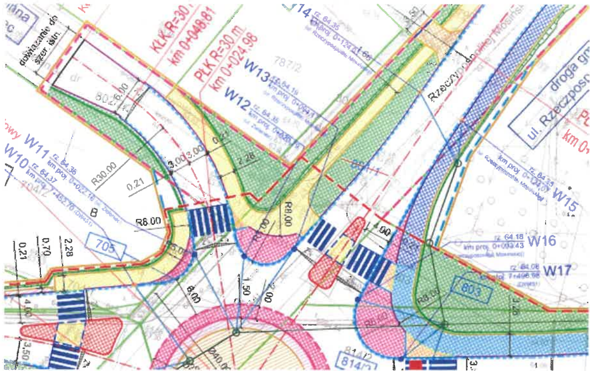
Rys. 1 wyrys z projektu budowy ronda w kierunku ul. Zieleniec - brak kontynuacji ścieżki
